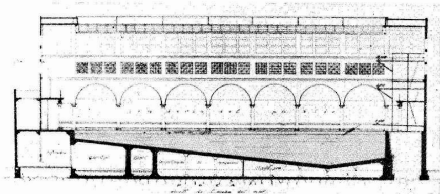
Sección longitudinal de la sala de la piscina
